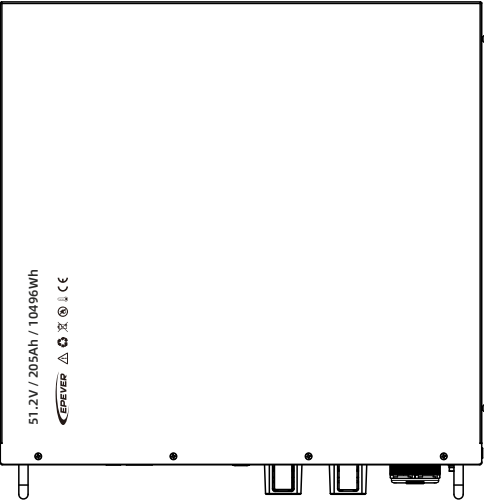
俯视图
