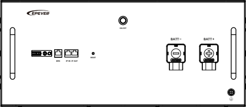
正视图
