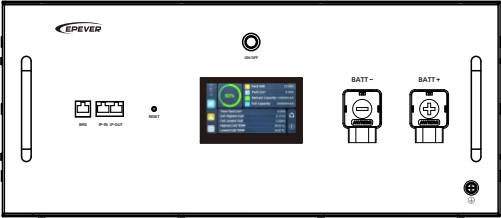
正视图
