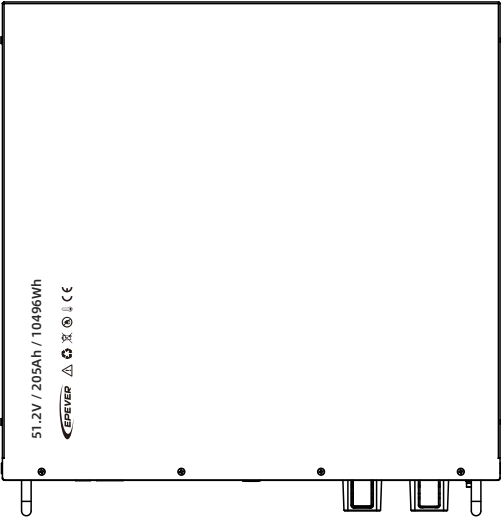
俯视图
