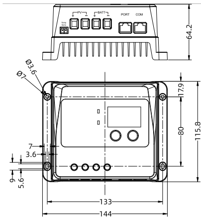
TRC3210
