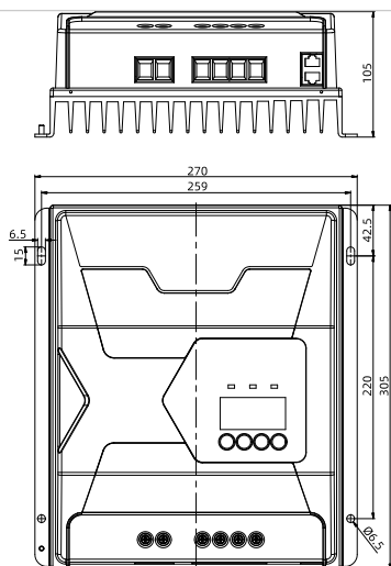
TIS7425 (单位: mm)
