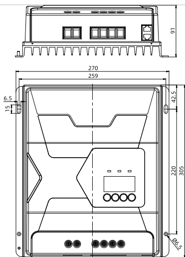
TIS8425/TIS10415 (单位: mm)
