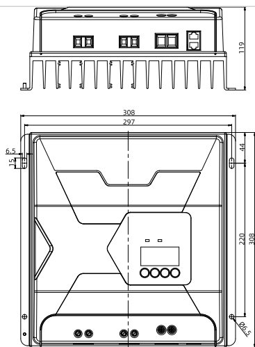
TES8425/TES10415 (单位: mm)
