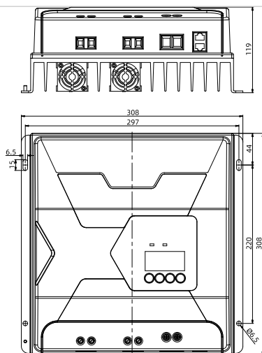
TES10425 (单位: mm)
