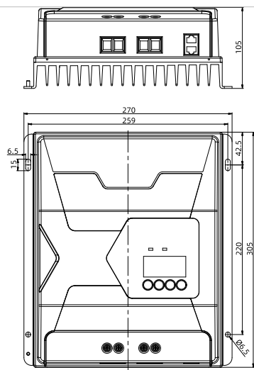
TES10425 (单位: mm)
