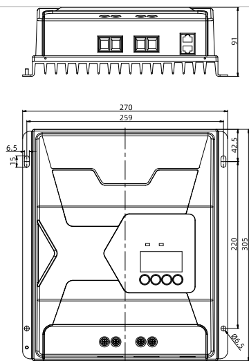
TES8425/TES10415 (单位: mm)
