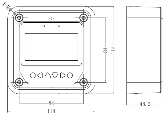
MT50 底壳安装尺寸
