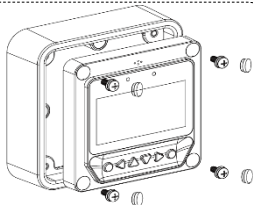
MT50 面板安装
