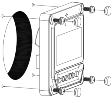
面板安装示意图
