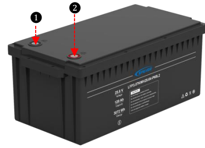
① 锂电池负极端子 ② 锂电池正极端子
