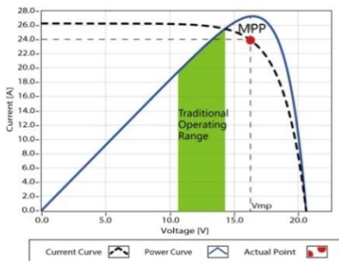
图 1-2 最大功率点跟踪曲线
