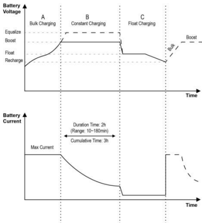
图 1-4 蓄电池充电阶段示意
