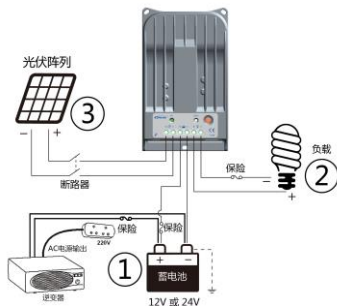
图 2-1 接线示意图
